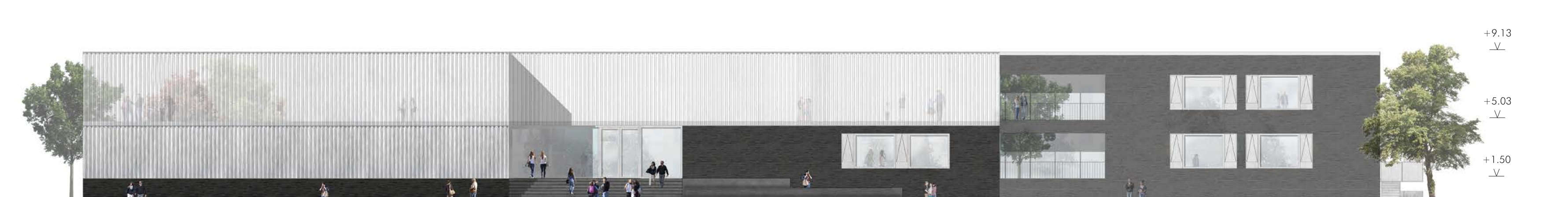
PROSPETTO OVEST - VIA GENOVA SCALA 1:200
