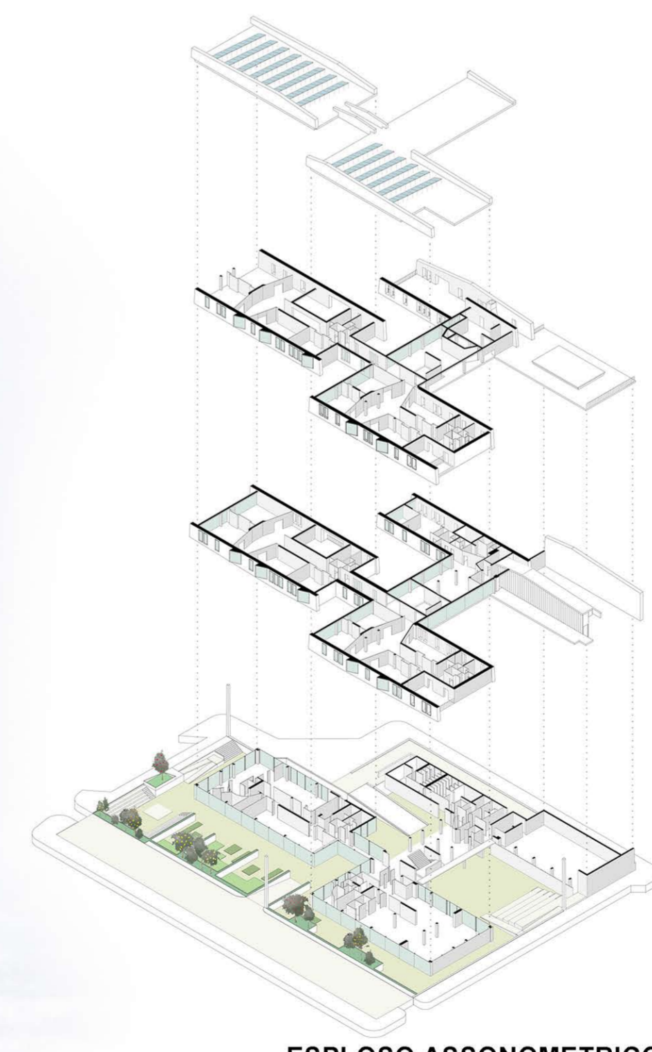
ESPLOSO ASSONOMETRICO
